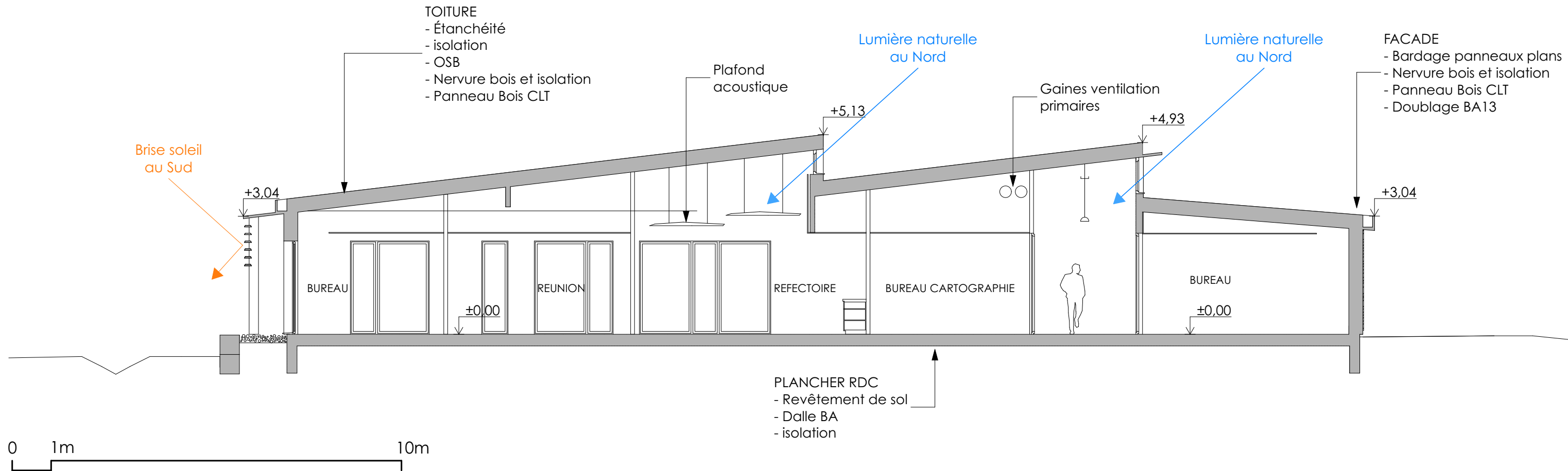
Coupe BB
