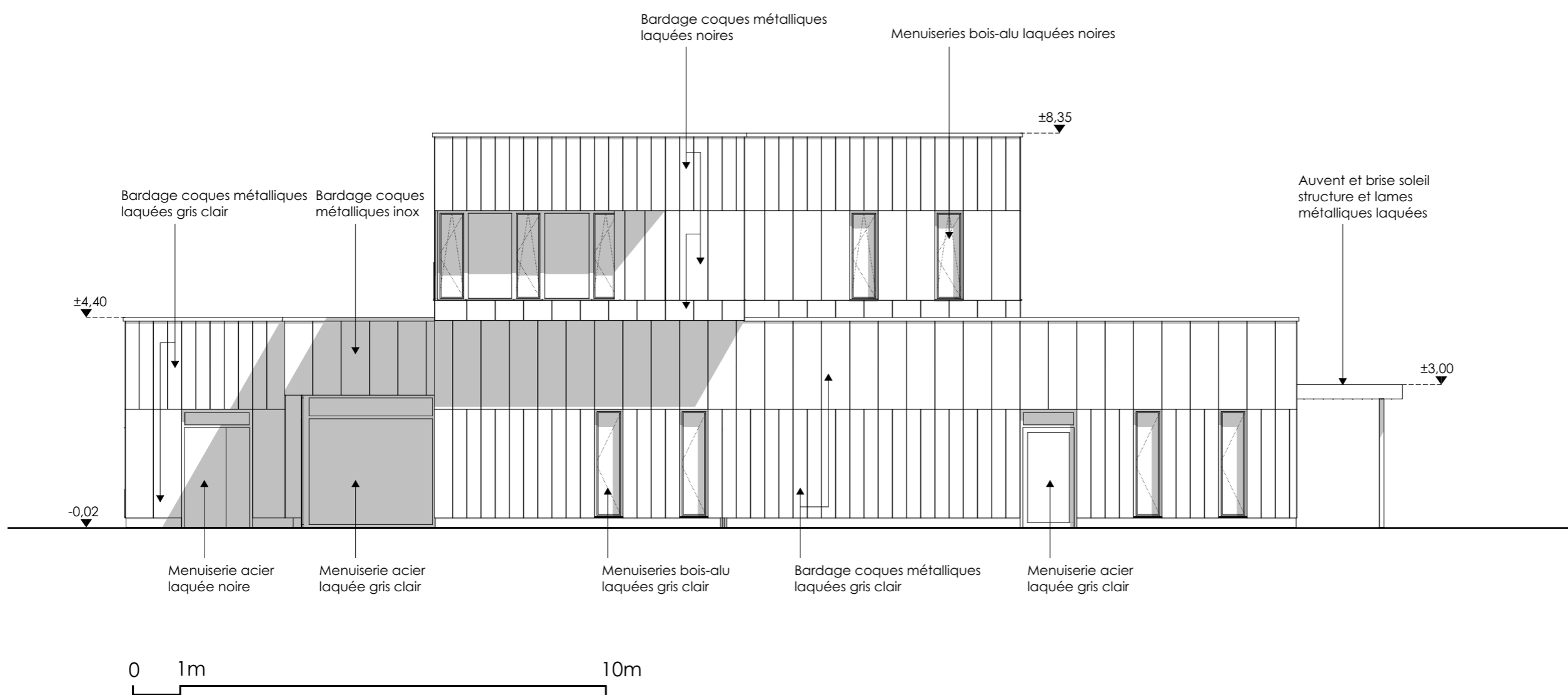
Elévation ouest - bâtiment administratif et technique
