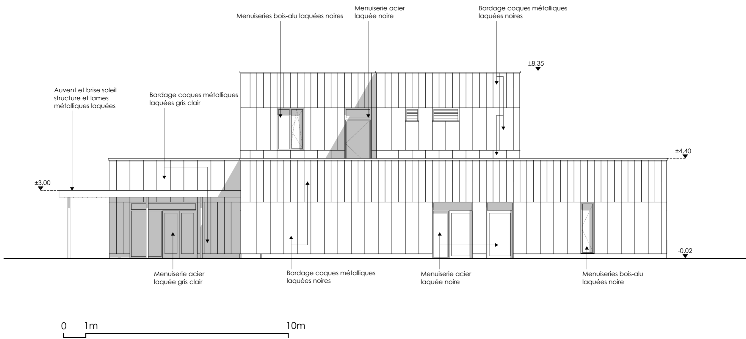
Elévation est - bâtiment administratif et technique
