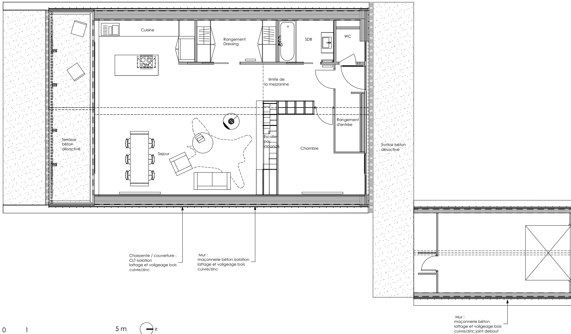
Plan RDC
